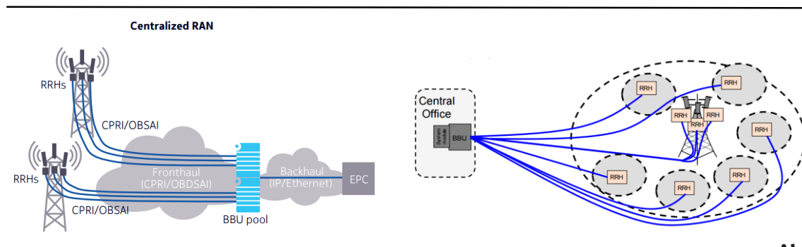
Abbildung 2-24: Gepoolte BBU mit breitbandiger Anbindung der RRH
