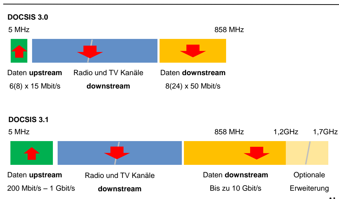
Abbildung 2-18: Typische Frequenzbelegung von DOCSIS 3.0 und 3.1 im Vergleich
