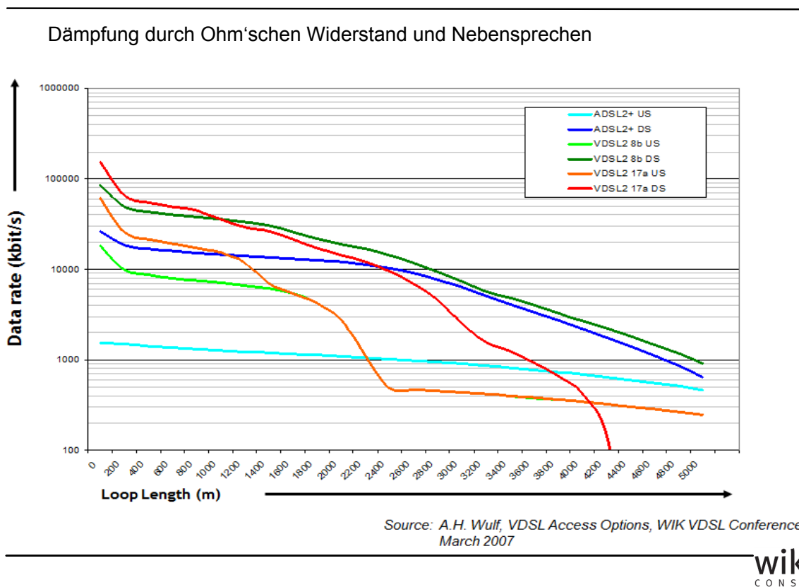
Abbildung 2-1: Übertragungsbandbreiten bei ADSL 2+ und VDSL2 über die Länge der Anschlussleitung
