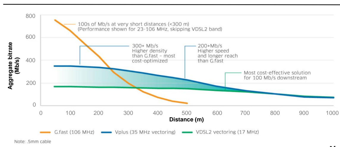
Abbildung 2-15: Bandbreiten von G.fast, VDSL Profil 35b und 17a im Vergleich über die Anschlussleitungslänge
