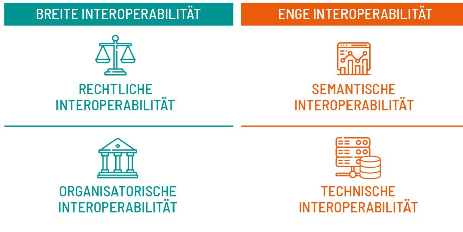
Grafik 4: Interoperabilitäts-Ebenen 83
