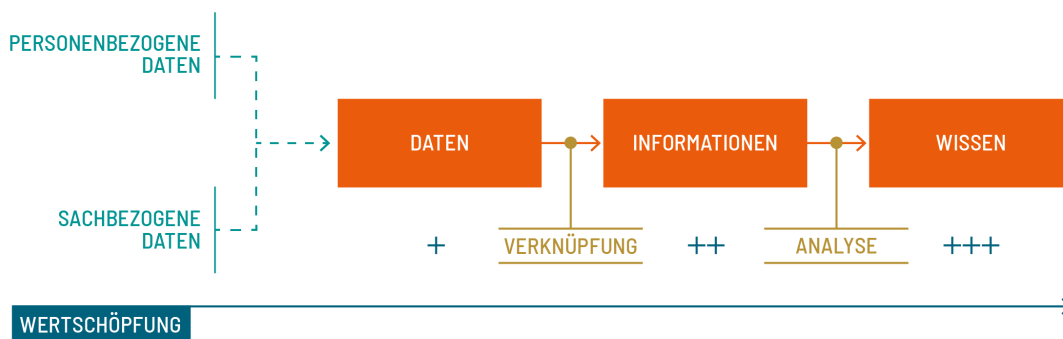
Grafik 1: Datenwertschöpfungskette 18
