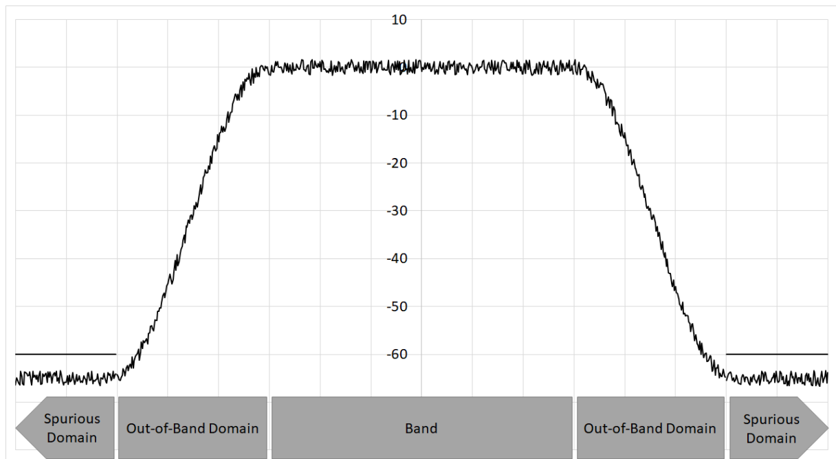
Illustration 1: Représentation graphique de la bande à brouiller, du domaine hors bande et du domaine des rayonnements non essentiels. Dans cet exemple, la bande à brouiller est inférieure à 1 GHz; pour de brefs engagements de brouillage (catégorie 2), une valeur limite de -60 dBc s'applique aux interférences émises non souhaitées dans le domaine des rayonnements non essentiels, sans que ces interférences doivent être inférieures à -36dBm ERP.
