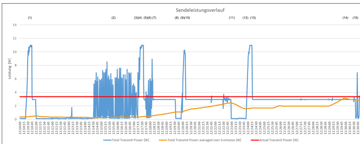
Abbildung 3: Sendeleistung während dem Ablauf des Downloads
