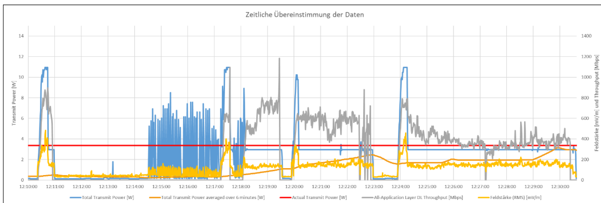
Abbildung 6: Zeitliche Übereinstimmung der Messdaten
